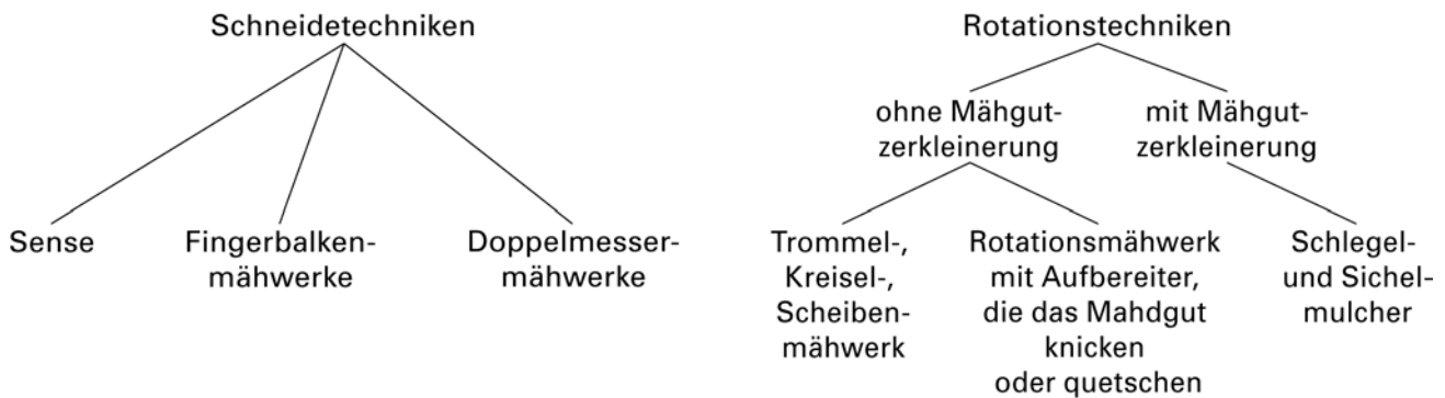
Abb. 2: Schematische Gliederung üblicher Mähtechniken anhand der Funktionsweisen.
